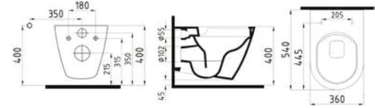
ASMA KLOZET NO-RİM ALKA054H1VP1W5000 540x360 mm
