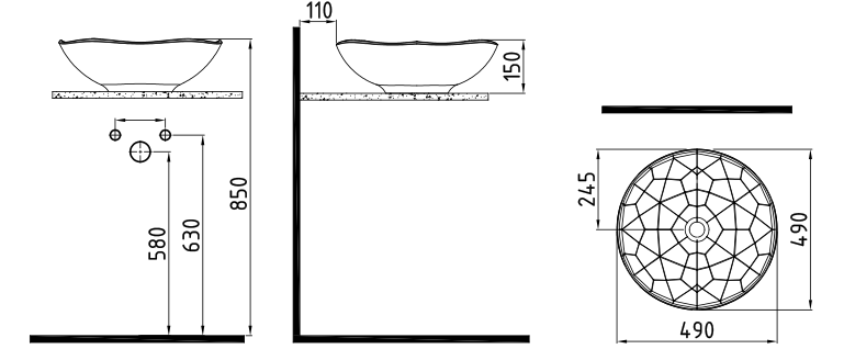
GÖVDE ÜSTÜ LAVABO BATARYA DELİKSİZ / TAŞMA DELİKSİZ PNLG04901FD0W5000 Ø490 mm
