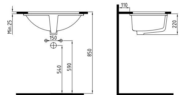
TEZGAHALTI LAVABO BATARYA DELİKSİZ ROSE GOLD DEKORLU TAŞMA DELİKLİ FALG05301FD009SZ00 550x325 mm Rose Gold Kaplama Beyaz TEZGAHALTI LAVABO BATARYA DELİKSİZ TAŞMA DELİKLİ FALG05301FD00W3SZ0 550x325 mm Beyaz
