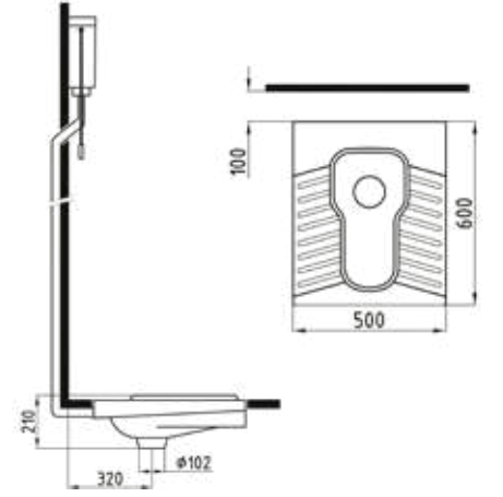
ÇEVRE YIKAMALI HELA TAŞI TPHT05002VSAW5000 500x600 mm Arkadan su girişli.
