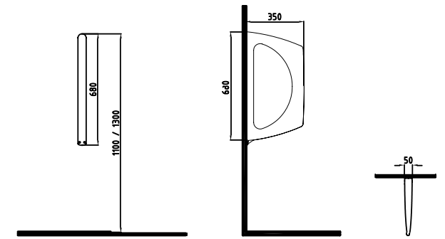
PİSUAR ARA BÖLME NPPA06801V00W5000 680x350 mm
